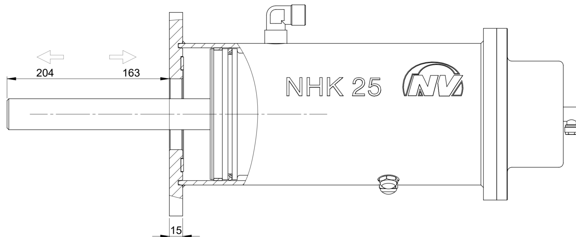
2 Version mit Bausatz-Stößel Version with rod kit
